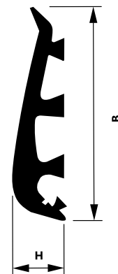
Fig.1: Muffenkonturprofil MKP-97 (mit SD-97) und plastomeres Lastübertragungsring CLE
